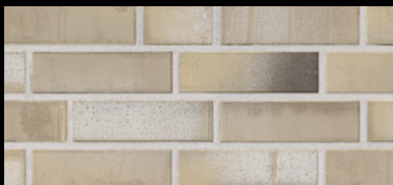
490 sandgrau Δ < 3 % · DIN EN 14411, Gr. A 1
