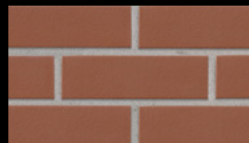
215 patrizierrot Δ < 3 % · DIN EN 14411, Gr. AII g
