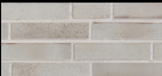
670 sandweiss Δ < 3 % · DIN EN 14411, Gr. A 1
