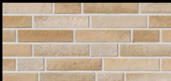
454 creme-weiß used look Δ < 3 % · DIN EN 14411, Gr. A 1
